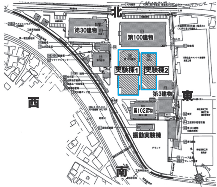
藤沢テクノセンター配置図（建替え後）
